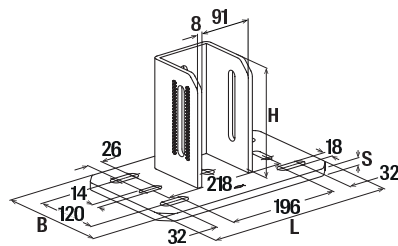
FMSF 120M
