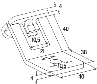
FSB 45°
